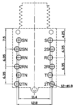
印制线路板示意图(底视图) P.C.B. Layout(Bottom View)
