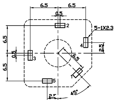
印制线路板示意图(底视图) P.C.B. Layout(Bottom View)
