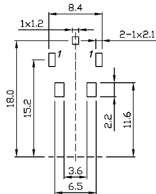
P.C.B LAYOUT(±0.1) (BOTTOM VIEW)
