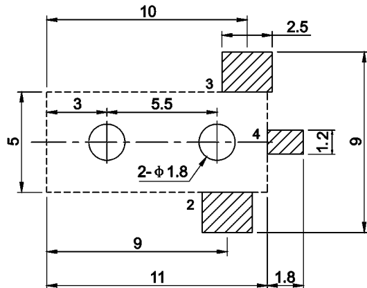
线路板印制示意图
