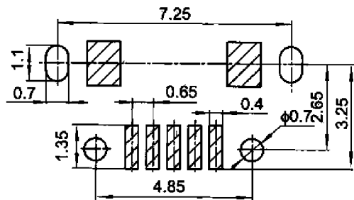
印制线路板推荐开孔尺寸
