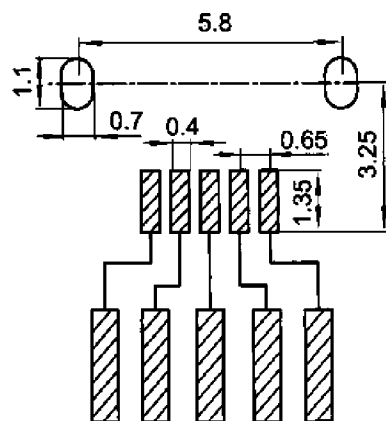
印制线路板推荐开孔尺寸
