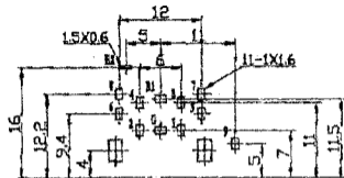
印制线路板开孔尺寸
