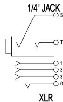
接点示意图 Schematic Layout
