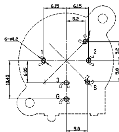
印制线路板示意图(底视图) P.C.B. Layout(Bottom View)
