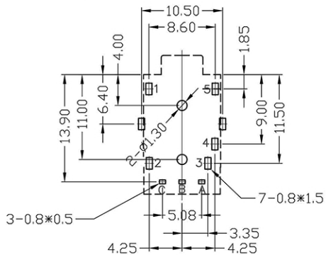
基板下參考圖(公差 \pm 0.3 ) PCB LAYOUT(Tol. \pm 0.3 )
