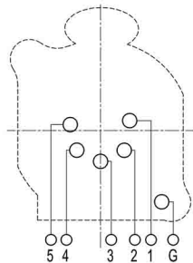
印制线路板示意图(底视图) P.C.B. Layout(Bottom View)
